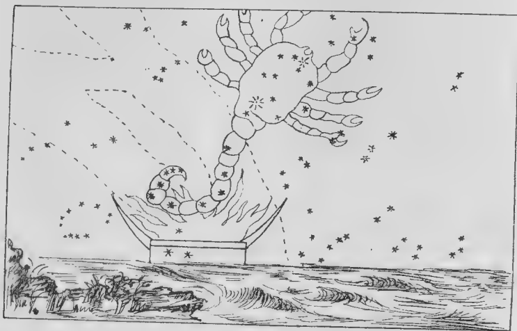
Рис. 25. Созвѣздіе Жертвенника на южномъ горизонтѣ Патмоса.
