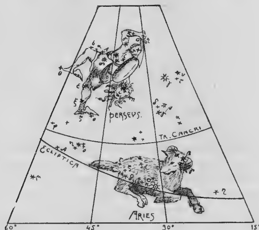
Рис. 50. Прохождение Овна черезъ меридианъ.
