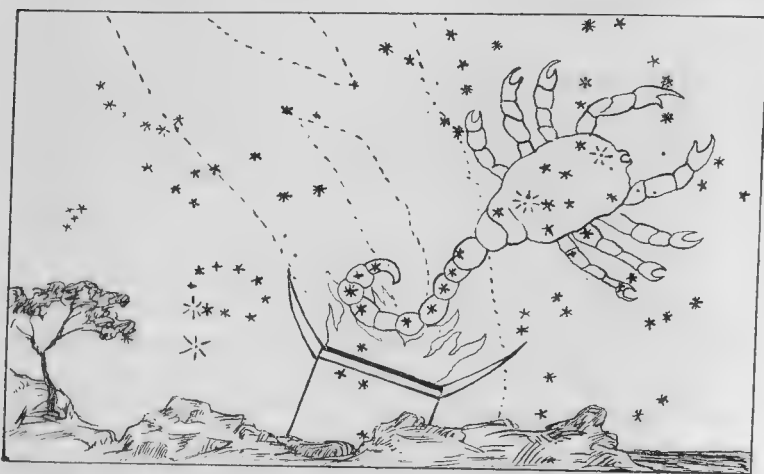
Рис. 30. Созвѣздіе Скорпіона и Жертвенника вечеромъ 30 Сентября 395 года.
