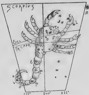
Рис. 26. Сатурнъ (♄) близъ челюстей Скорпіона, въ его головогрудѣ, 30 сентября 395 года.
