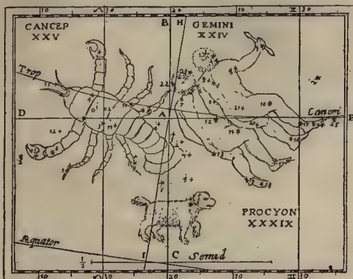
Созвѣдія: Ракъ и Близнецы.
