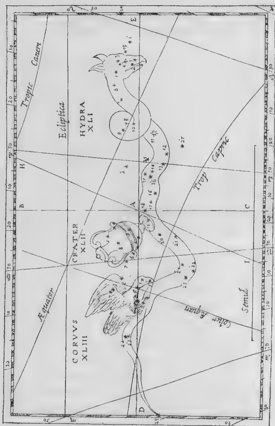
Рис. 52. Созвѣздіе Самка Гидры и Чаша.
