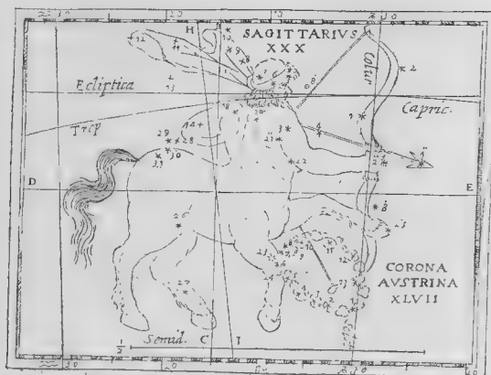
Рис. 20. Созвѣздіе Стрѣльца, гдѣ солнце бываетъ въ началѣ зимы, по Griemb.
