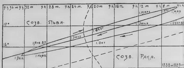
Рис. 4. Путь Сатурна между созвѣздіями Рака и Льва въ 1888 и 1889 гг.
