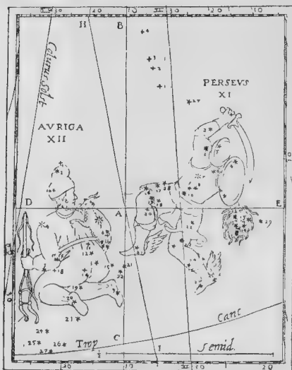
Рис. 45. Созвѣздія Возничаго Конскихъ Уздъ и Персея (по Гринбергеру, 1612 г.).
