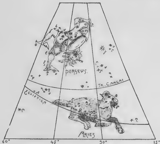
Рис. 24. Марсь (♂) 30 сентября 395 года въ срединѣ Овна подъ мечемъ Персея.
