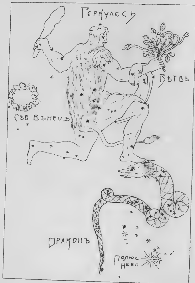
Рис. 35. Созвѣздіе Геркулеса, избивающаго змѣй дубиной (По манускр. Гринбергера въ Пулк. обсерв.).
