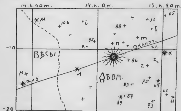
Рис. 58 Положеніе солнца въ созвѣздіи Дѣвы для 30 сентября 395 юліанскаго года.
