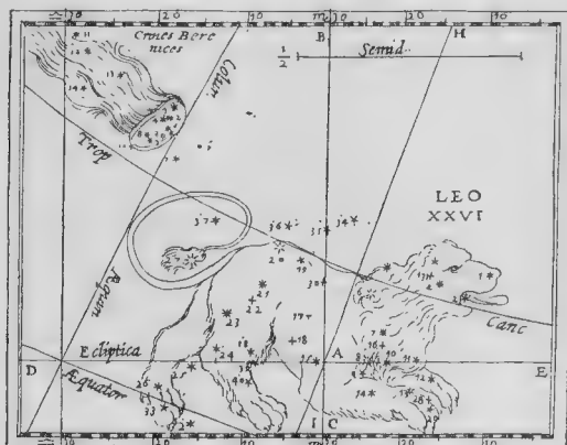
Рис. 18. Созвѣздіе Льва, гдѣ солнце бываетъ передъ началомъ осени, по Grienberger'у.
