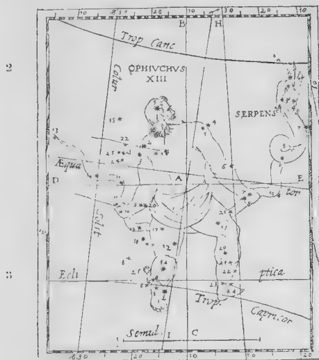
Рис. 53. Созвѣздіе Зміеносца, съ небеснымъ экваторомъ, опоясывающимъ видимый сводъ.
