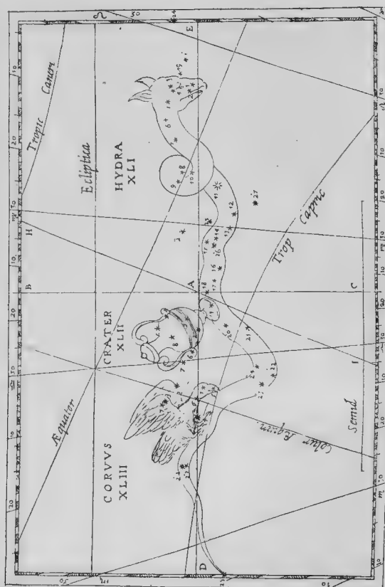
Рис. 49. Созвѣздіе Самка Гидры и Чаша.
