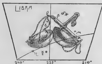
Рис. 25. Положеніе невидимаго Меркурія (♿) въ Вѣсахъ 30 сентября 395 года.
