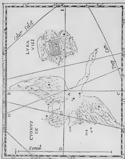
Рис. 46. Созвѣздіе Лебедя и Лирь (по атласу Гринбергера, 1612 г.)
