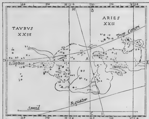
Рис. 19. Созвѣздіе Тельца, гдѣ солнце бываетъ пе- редъ началомъ лѣта, по Grienberger'у.
