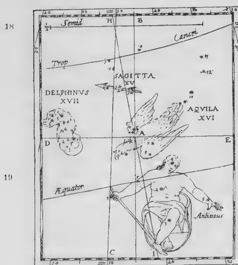
Рис. 51. Созвѣздіе Орла, Дельфина и Антиная (по Гринбергеру).
