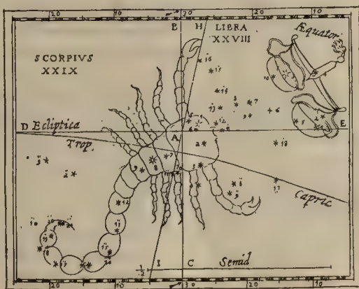
Созвѣдія: Вѣсы и Скорпіонъ.
