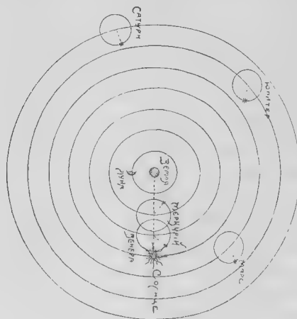
Фиг. 62. Система Птолемея (половина 2-го вѣка).
