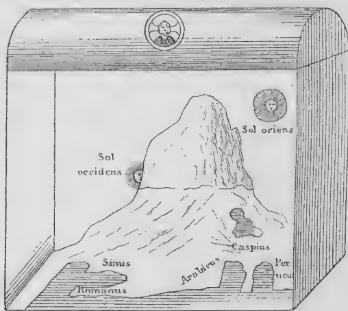
Рис. 56 Вселенная древнихъ христіанъ изъ Cosmas Indicopleustes, 535 г.
