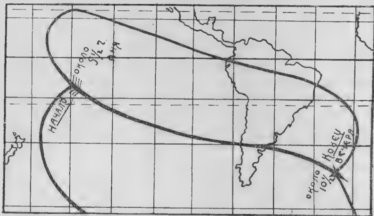
Рис. 61. Путь солнечнаго затменія 30 сентября 395 г. по Патмосскому времени.
