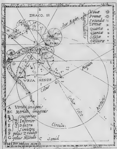
Рис. 36. Созвѣздіе Дракона, по манускрипту Гринбергера въ Пулк. Обсерв.
