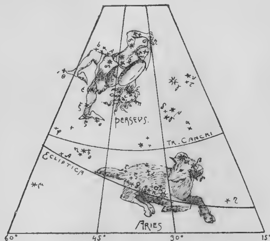
Рис. 59. Марсъ подъ Персеемъ въ Овнѣ.
