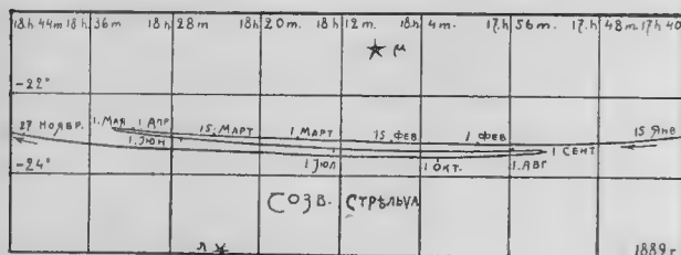
Рис. 5. Путь Юпитера по созвѣздію Стрѣльца въ 1889 г.
